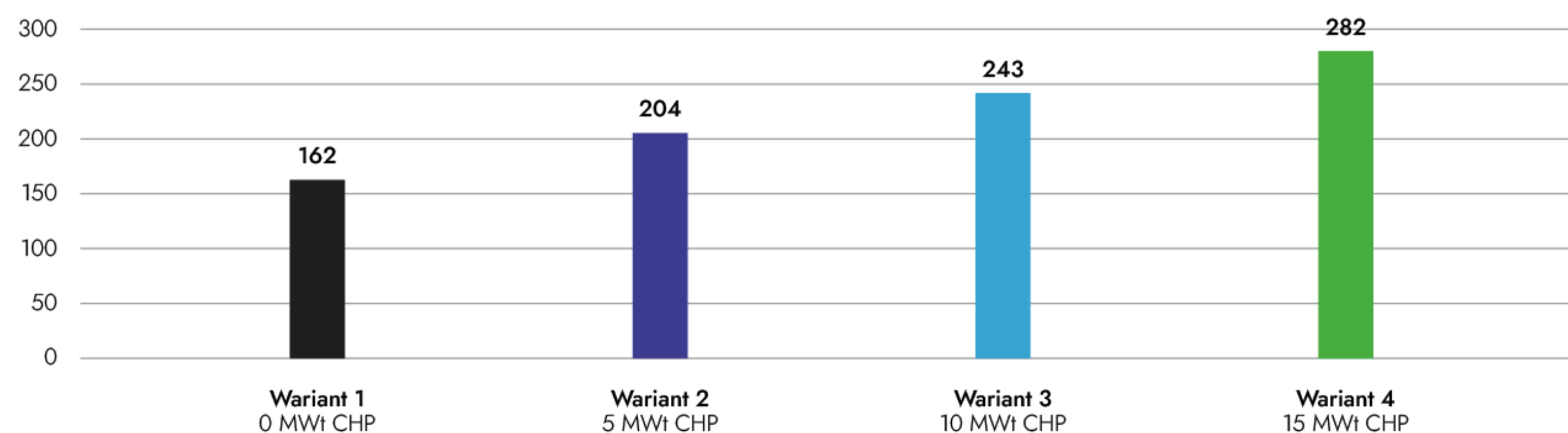
CAPEX nominalnie [mPLN] Rynek 35 MW
