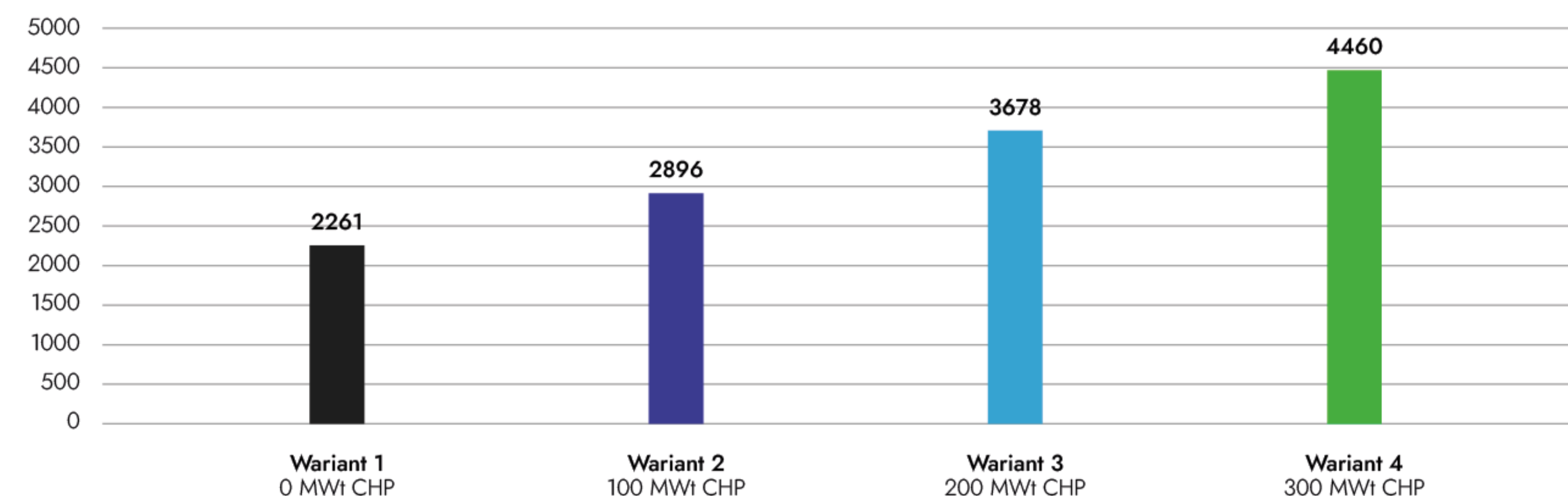
CAPEX nominalnie [mPLN] Rynek 600 MW
