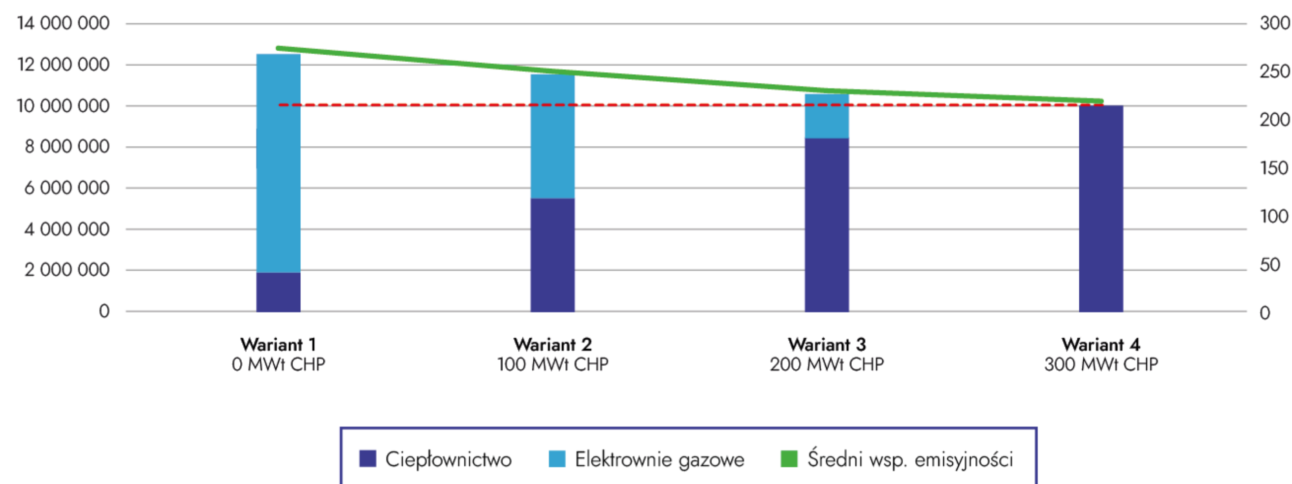
Łączna emisyjność CO 2 [tCO 2 ] oraz średni współczynnik emisyjności [g/kWh] dla systemu ciepłowniczego i elektroenergetycznego w latach 2030-2044, rynek 600 MW
