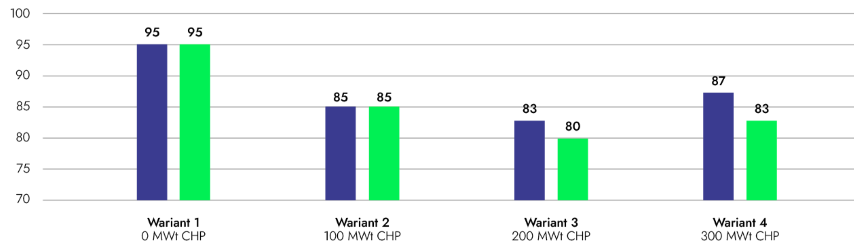
LCOH [PLN'25/GJ] Rynek 600 MW
