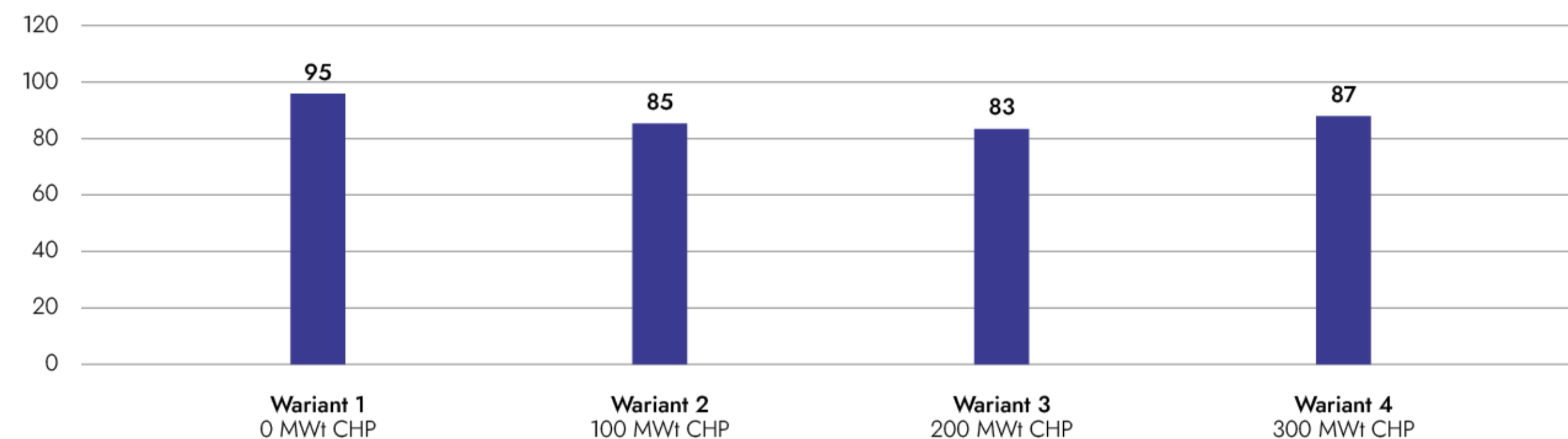
LCOH [PLN'25/GJ] Rynek 600 MW
