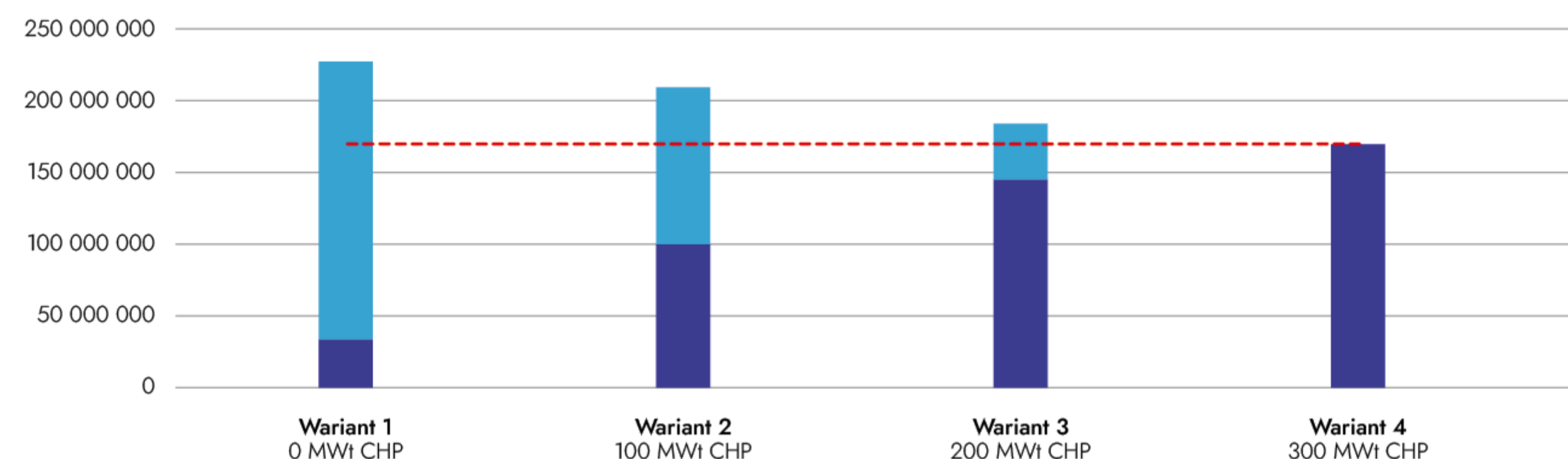
Łączne zużycie gazu [Gj] dla systemu ciepłowniczego i elektroenergetycznego w latach 2030-2044, rynek 600 MW
