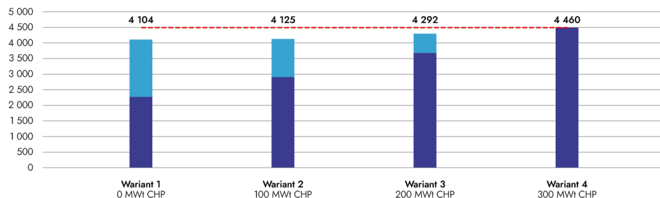
CAPEX nominalnie [mPLN], rynek 600 MW
